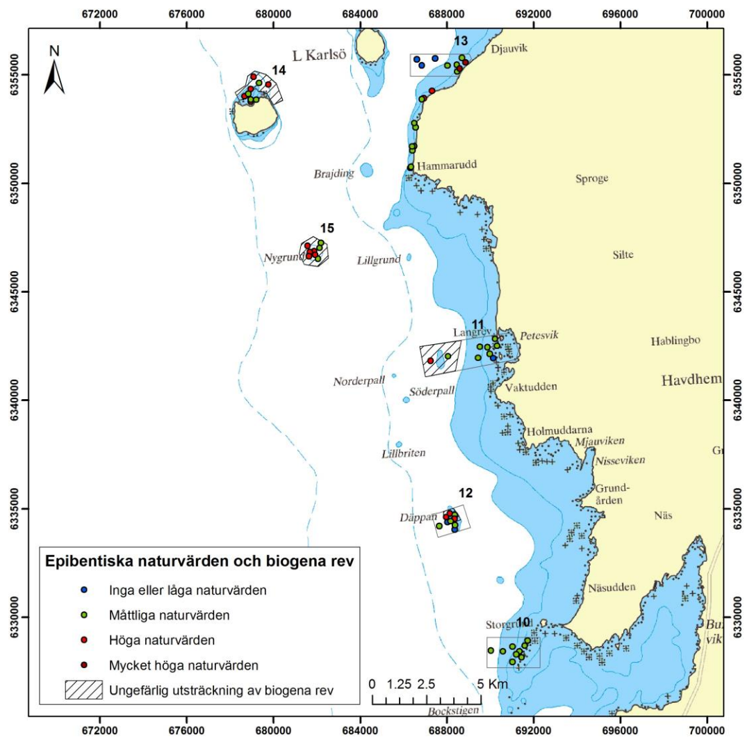
Figur 30. Epibentiska naturvärden samt ungefärlig utsträckning av biogena rev i undersökta områden utanför Gotlands södra västkust.
