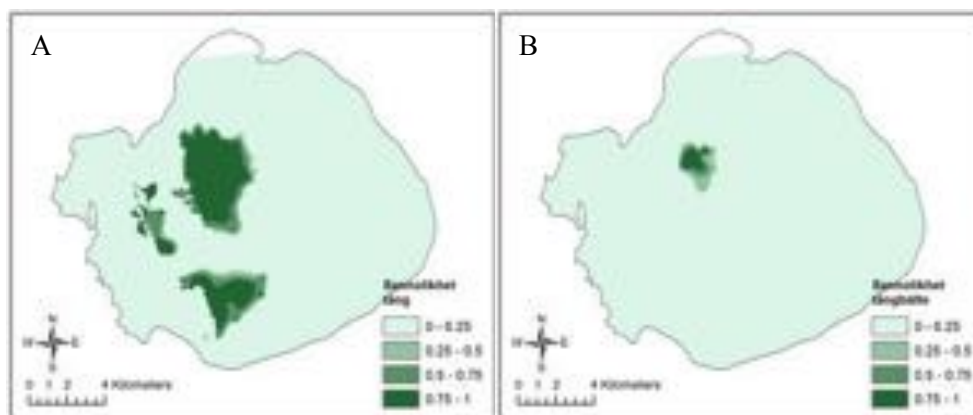
Figur 9 Sannolikheten för förekomst av tang (A) och tangbälte (B) på Finngrundet Östra banken. Områdets yttre begränsning sammanfaller med tidigare föreslagna gränsen för grundet, vilken motsvarar gränsen för 30 m djup.
