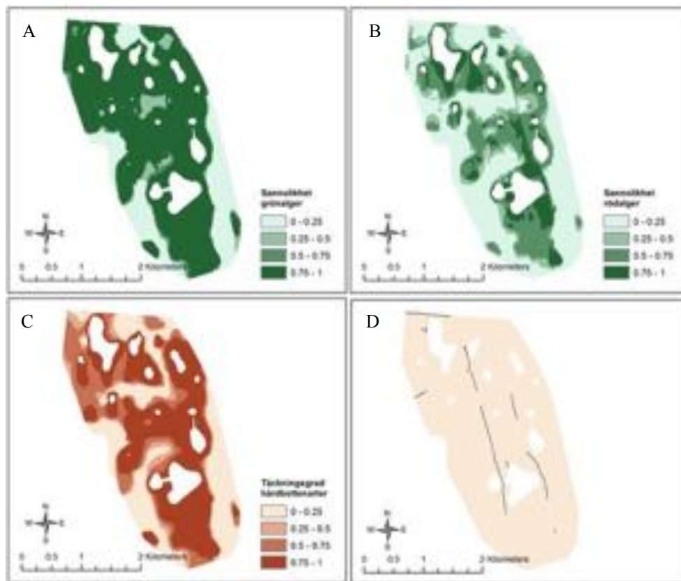
Figur 7. Sannolikheten för förekomst av modellerade alger (A-B), täckningsgrad av samtliga hårbottenarter (C) samt videotransekterna (D) på Väktaren. De vita ytorna utgör områden med mindre än 3 m djup, där det inte fanns några inventeringsdata.
