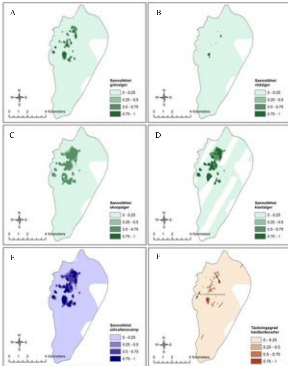
Figur 6. Sannolikheten för förekomst av de modellerade algerna (A-D) och sötvattenssvamp (E) samt täckningsgrad av samtliga hårdbottenarter (F) på Rata Storgrund. Prediktionen för kiselalger, där bottensubstrat var en viktig faktor i modellen, visas bara för de transekter där det finns information om bottensubstratet. De grå linjerna visar den yttre gränsen för grundet enligt den tidigare rapporten från utsjöbanksinventeringen (Naturvårdsverket 2006) och motsvarar djupkurvan för 19 m djup. Videotranskterna är inlagda i delfigur F.
