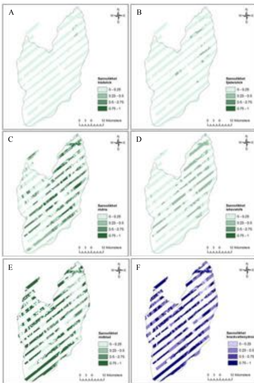
Figur 10. Sannolikheten för förekomst av modellerade makroalger (A-E) och bräcksvattenhydroiden C. caspia (F) på Hoburgs Bank. Den grå heldragna linjen visar den föreslagna yttre begränsningen för grundet.
