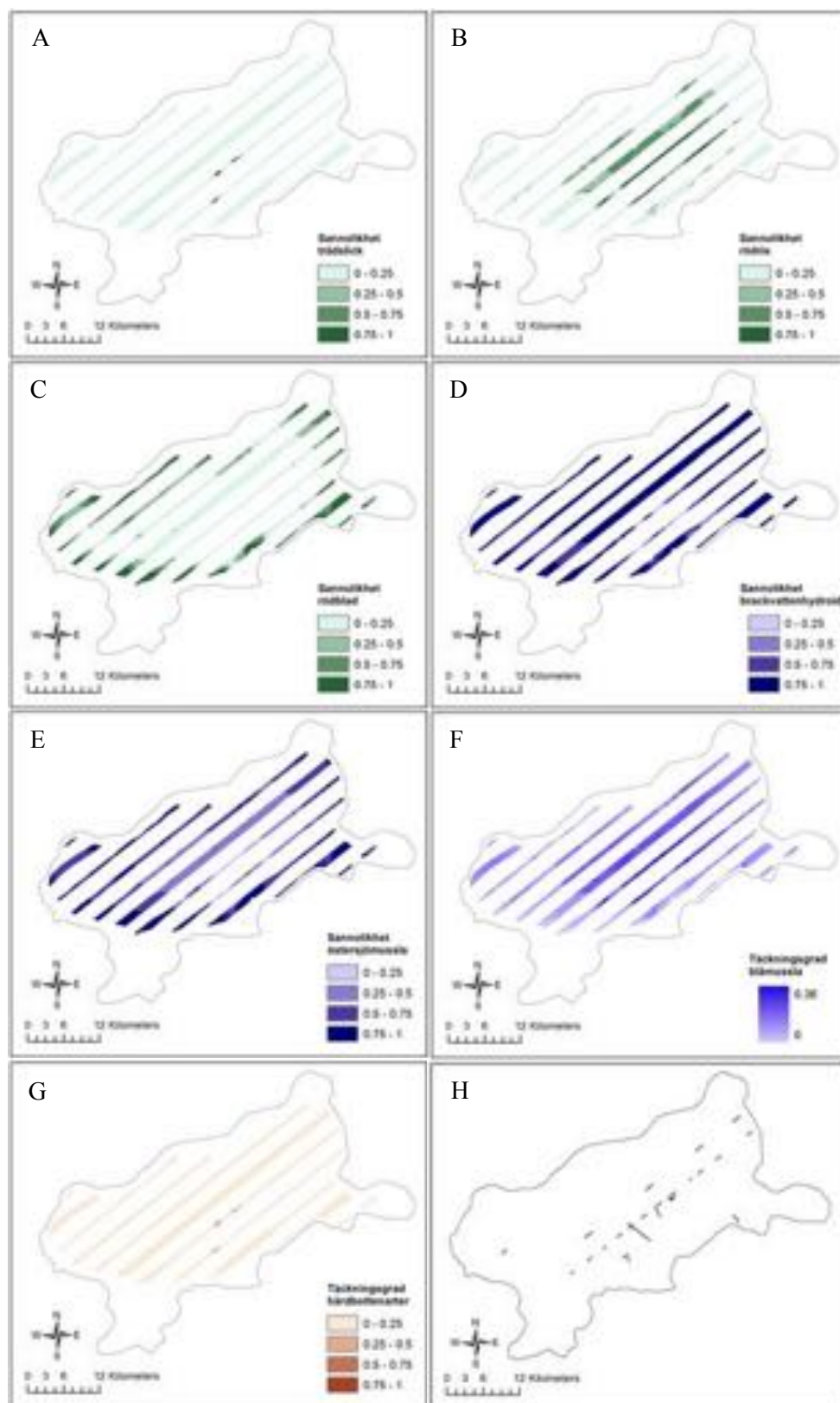
Figur 11. Sannolikheten för förekomst av några modellerade makroalger (A-C) och djur (D-E), täckningsgrad av blåmussla (F) och samtliga hårdbottenarter (G), samt videotranssekterna (H) på Norra Midsjöbanken. Den grå heldragna linjen visar den föreslagna yttre begränsningen för grundet. Observera att skalan för täckningsgrad av blåmussla skiljer sig från övriga delfigurer.
