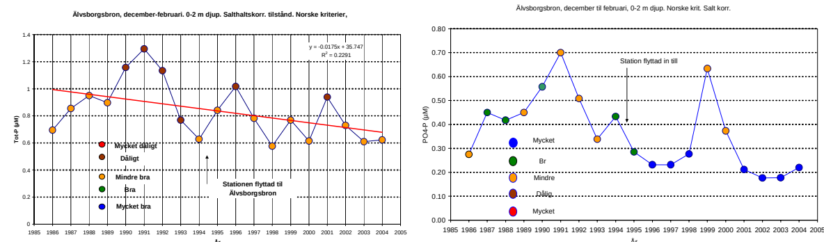
Figur 31. Vintervärden (dec-feb) för tot-P och PO 4 -P i ytvattnet (0-2 m) vid Älvsborgsbron 1986-2004 (µM) jämförda med norska kriterier för miljöklassning (Molvær m fl 1997). Värdeklasserna är korrekterade för salthalten. Pilen markerar när mätstationen flyttades till öster om Älvsborgsbron 1994.
