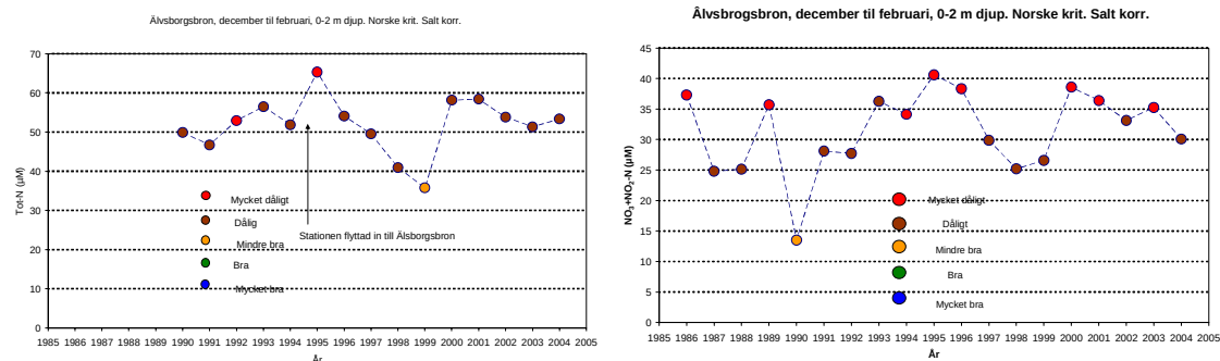
Figur 32. Vintervärden (dec-feb) för totalkväve och nitrit plus nitratkväve ( \text{NO}_x\text{-N} ) i ytvattnet (0-2 m) vid Älvsborgsbron 1990/86-2004 ( \mu\text{M} ) jämförda med norska kriterier för miljöklassning (Molvær m fl 1997). Värdeklasserna är korrigerade för salthalten. Pilen markerar när mätstationen flyttades till öster om Älvsborgsbron 1994
