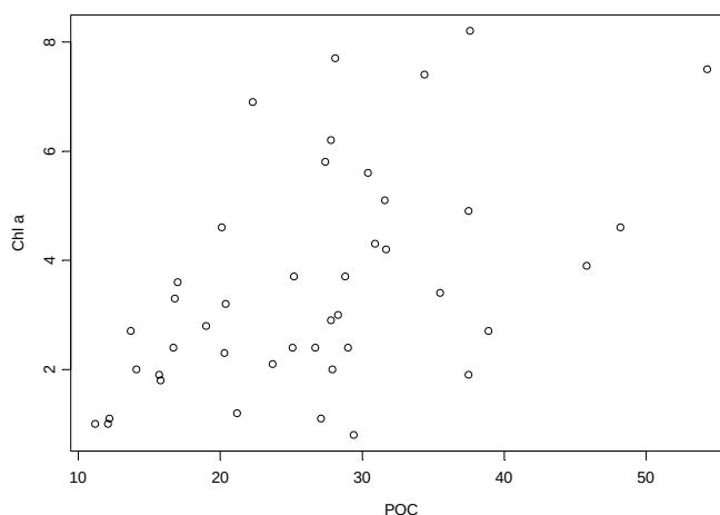
Figur 20. Partikulärt organisk kol (POC) korrelerar signifikant med klorofyll a i ytvattnet i Danafjord. Data från Bohuskustens kontrollprogram 1997-2004.
