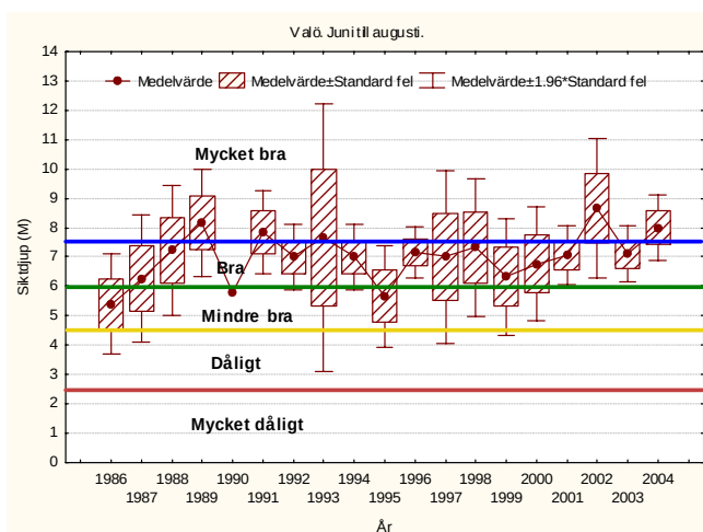
Figur 26. Mätvärden för siktdjupet under sommaren (jun-aug) vid Valö 1986-2004 (µM) jämförda med norska kriterier för miljöklassning (Molvær m fl 1997).
