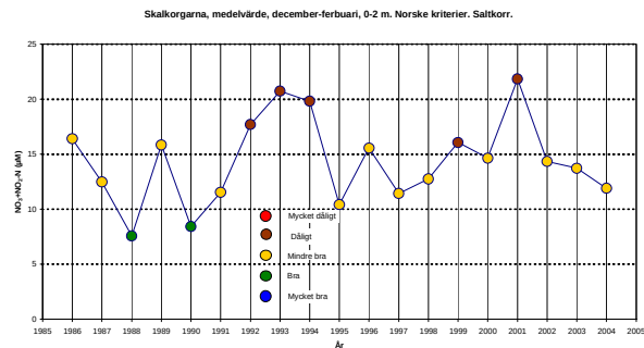
Figur 28. Mätvärden för totalkväve och nitrit plus nitratkväve ( \text{NO}_x\text{-N} ) i ytvattnet (0-2 m) vid Skalkorgarna 1986/90-2004 ( \mu\text{M} ) jämförda med norska kriterier för miljöklassning (Molvær m fl 1997). Värdeklasserna är korrigerade för salthalten. Vintervärden, dec-febr.
