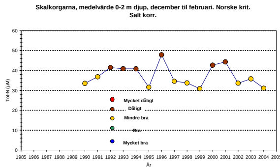
Figur 28. Mätvärden för totalkväve och nitrit plus nitratkväve ( \text{NO}_x\text{-N} ) i ytvattnet (0-2 m) vid Skalkorgarna 1986/90-2004 ( \mu\text{M} ) jämförda med norska kriterier för miljöklassning (Molvær m fl 1997). Värdeklasserna är korrigerade för salthalten. Vintervärden, dec-febr.
