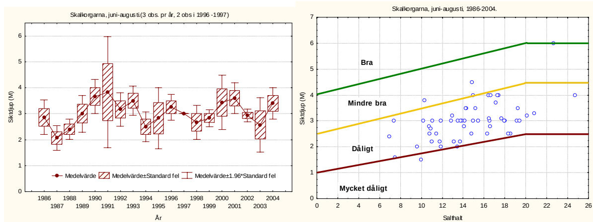
Figur 30. Till vänster mätvärden för siktdjupet vid Skalkorgarna 1986-2004 (µM). Till höger är samma data plottade mot salthalt och jämförda med norska kriterier för miljöklassning (Molvær m fl 1997). Sommarvärden, jun-aug.
