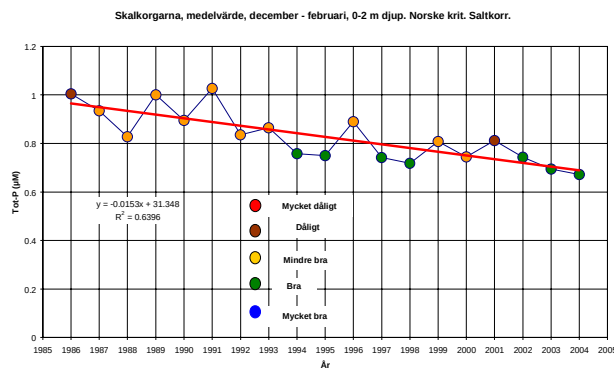
Figur 27. Mätvärden för tot-P och \text{PO}_4\text{-P} i ytvattnet (0-2 m) vid Skalkorgarna 1986/88-2004 ( \mu\text{M} ) jämförda med norska kriterier för miljöklassning (Molvær m fl 1997). Värderingarna är korrigerade för salthalten. Vintervärden, dec-febr.
