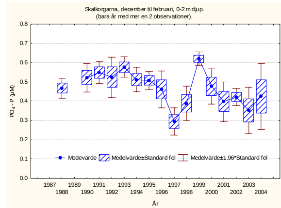
Figur 27. Mätvärden för tot-P och \text{PO}_4\text{-P} i ytvattnet (0-2 m) vid Skalkorgarna 1986/88-2004 ( \mu\text{M} ) jämförda med norska kriterier för miljöklassning (Molvær m fl 1997). Värderingarna är korrigerade för salthalten. Vintervärden, dec-febr.
