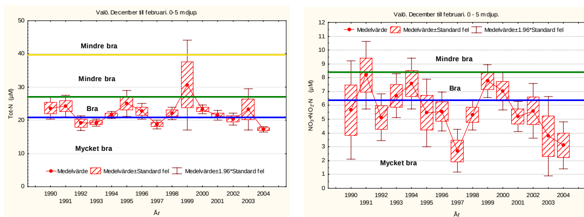
Figur 24. Mätvärden för totalkväve och nitrit plus nitratkväve (NO x -N) i ytvattnet (0-5 m) vid Valö 1990-2004 (µM) jämförda med norska kriterier för miljöklassning (Molvær m fl 1997). Vintervärden, december-februari.
