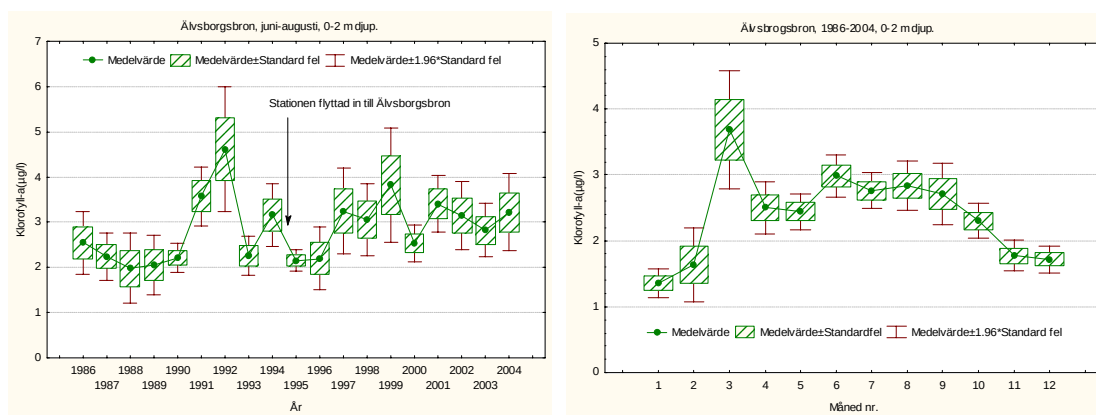
Figur 33. Sommarvärden (jun-aug) för klorofyll a i ytvattnet (0-2 m) vid Älvsborgsbron 1986-2004 ( \mu\text{M} ). Pilen markerar när mätstationen flyttades till öster om Älvsborgsbron 1994. Till höger variationen av klorofyll a över året.
